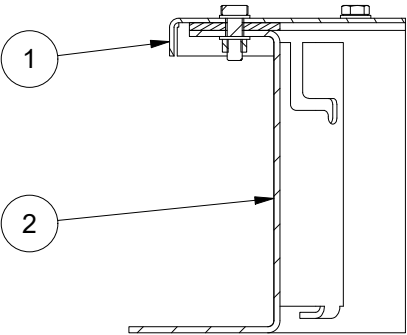
F-F ( 1 : 5 )
